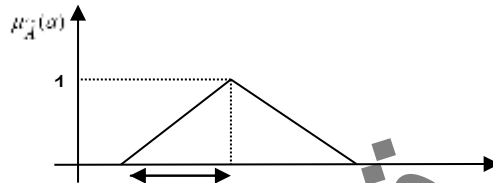
نمودار 1. عدد مثلثی \tilde{A} ماخذ: (تاناکا و همکاران، 1992) Figure 1. Fuzzy triangular number \tilde{A} Source: (Tanaka et al, 1992)
