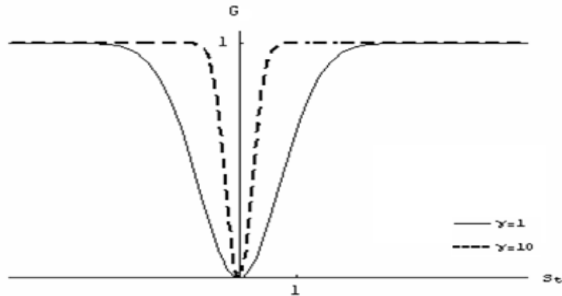
نمودار ۳. نمودار تابع انتقال نمایی مأخذ: (Teräsvirta, 1994)
