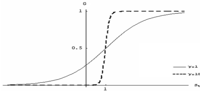
نمودار ۱. تابع لاجستیک با یک بار تغییر فاز مأخذ: (Teräsvirta, 1994)
